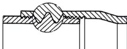
PVC Trapezoidal Threads DIN 4925
